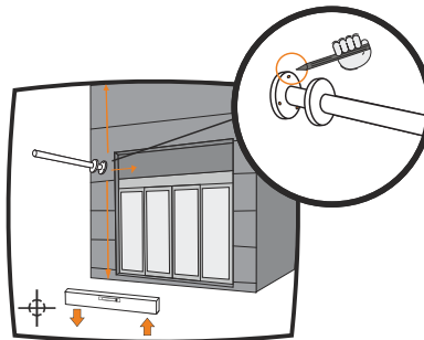
1.- Posicione el soporte nivelado y marque los tres agujeros
