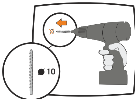
3.- Practique los agujeros indicados anteriormente sobre la pared.
