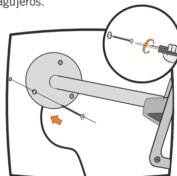
5.- Atornillar el foco a la pared.
