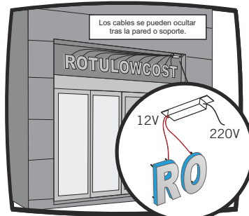
8.- Una vez colocadas todas, conectar cada letra al transformador led a través del cable lateral.
