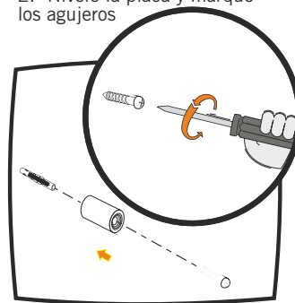
5.- Prepare el tornillo con la base del embellecedor (separador), como indica el dibujo
