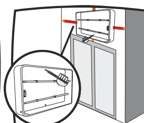
3. Marque los agujeros centrales sobre la pared, centrando el rótulo.
