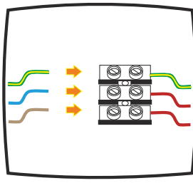
9. Realice la conexión eléctrica haciendo coincidir la línea de tierra.
